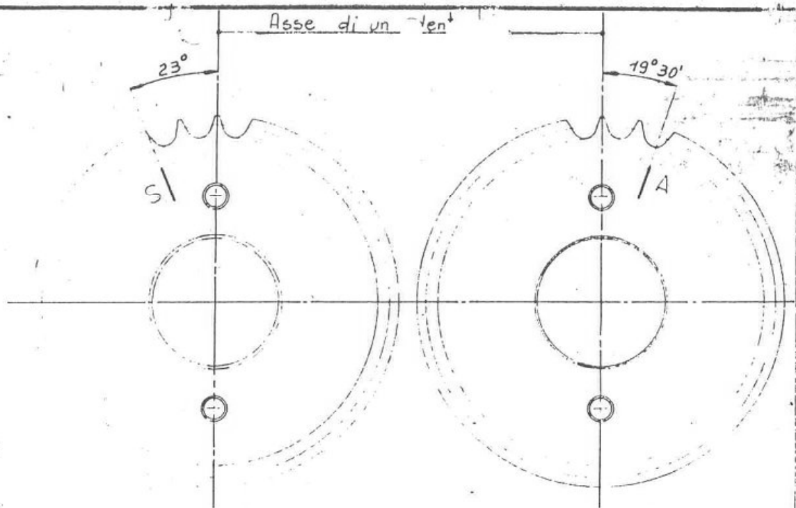
Corona comando albero a cammes di scarico (stampigliata) 41211110
